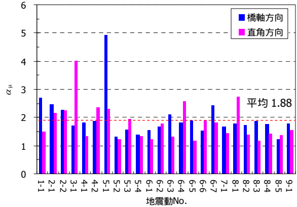
図-19 最大応答塑性率の最大値 / 最小値
