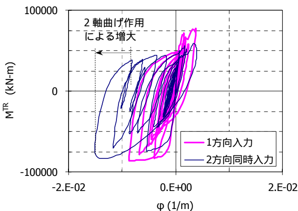
(b)橋脚基部のM - 履歴（橋軸回り）
