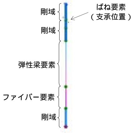
図-2 解析モデル図
