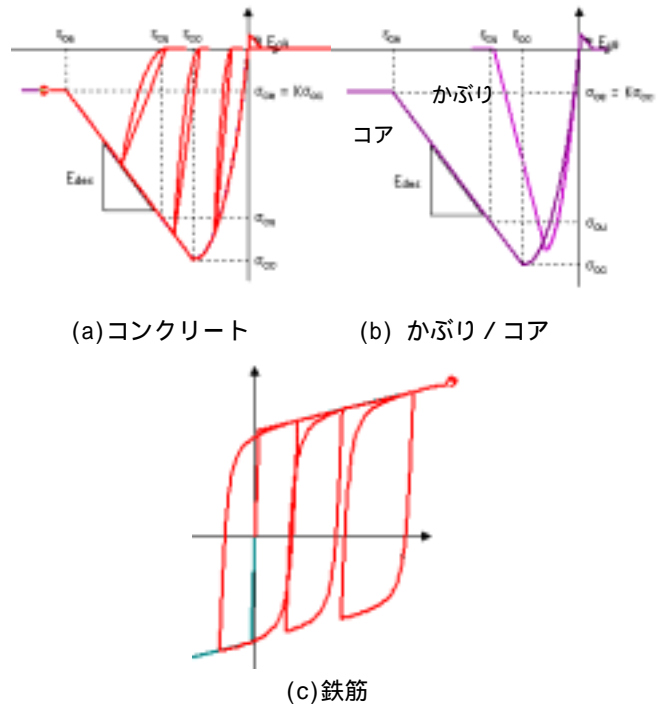
図-4 ファイバー要素に適用する材料履歴モデル
