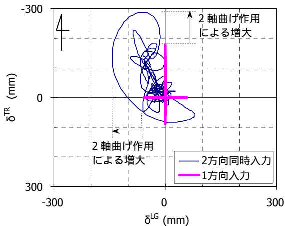
(a)橋脚天端の応答変位の軌跡
