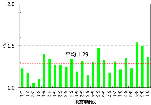
図-20 最大圧縮ひずみの最大値 / 最小値
