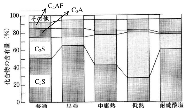
図 2.7 ポルトランドセメントの種類 1)
