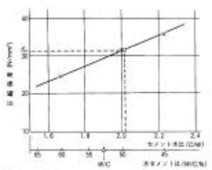
図 5.3 圧縮強度とセメント水比 (水セメント比) との関係の例
