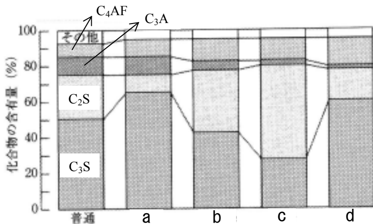
図 2.7 ポルトランドセメントの種類
