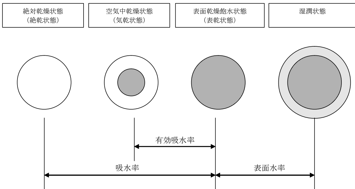
図 骨材の湿潤状態の説明
