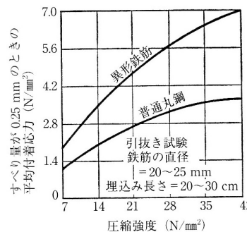
図4.13 付着強度と圧縮強度の関係 2)
