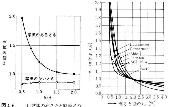
図 4.41 円柱供試体の高さとの径との比と強度との関係
