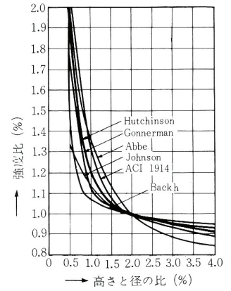
図 4.41 円柱供試体の高さ h と直径 d の比と強度との関係
