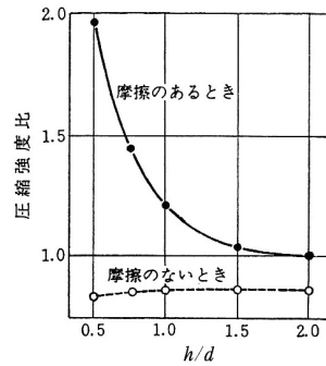
図 4.6 供試体の高さ h と直径 d の比と圧縮強度との関係 9)
