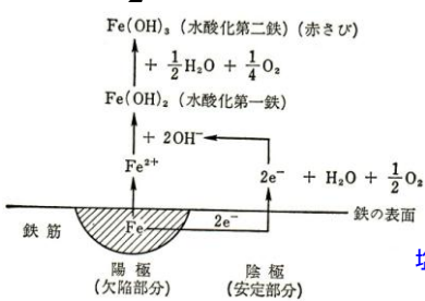
図 4.1 鉄筋の腐食反応機構
