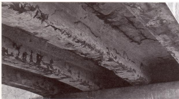
塩害で劣化した橋桁 かぶりコンクリートが剥落し、鉄筋が露出している。
