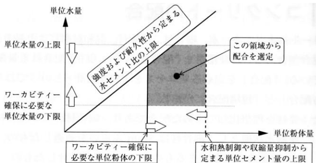
図 2・15 配合選定の考え方 (土木学会：「コンクリート標準示方書【施工編】(2007年制定)」, p.68 (解説図 4.1.1), (2008.3))
