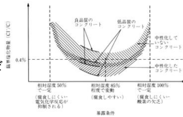
図 3.15 湿度とコンクリート品質が塩化物イオン量へ与える影響 (Schiesl 1985, FIP 1991)
