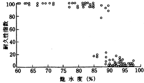
図-3 飽水度が耐凍害性に及ぼす影響
