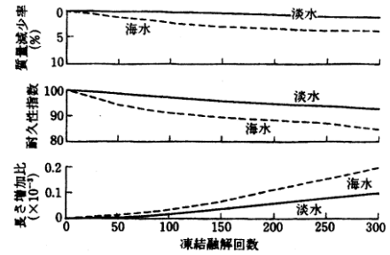
図-4 海水中と淡水中の凍結融解試験結果
