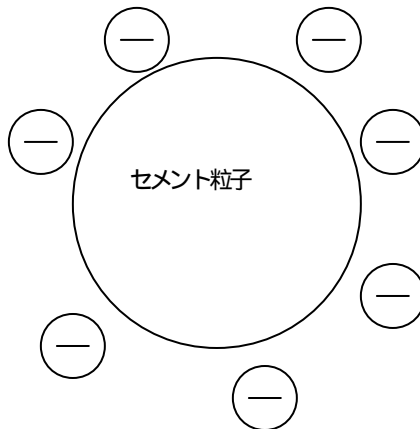
図 静電的な分散作用
